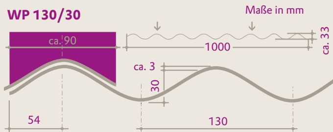
Querschnitt der PLEXIGLAS® Resist WP 130/30 (Maße in mm)
