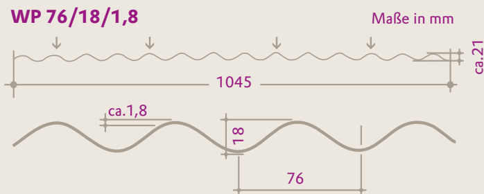
Querschnitt der PLEXIGLAS® Resist WP 76/18/1,8 (Maße in mm)
