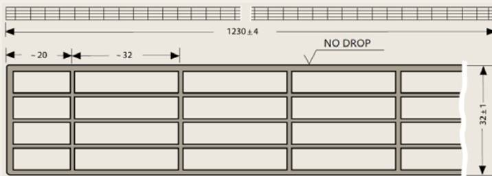
Querschnitt der PLEXIGLAS® Heatstop Cool Blue S5P 32 (Maße in mm)
