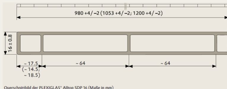
Querschnittsbild der PLEXIGLAS® Alltop SDP 16 (Maße in mm)
